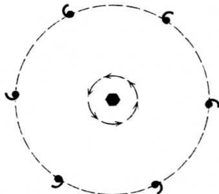
Rotation 60^\circ 6
