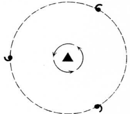
Rotation 120^\circ 3
