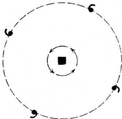
Rotation 90^\circ 4
