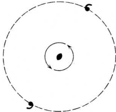
Rotation 180^\circ 2
