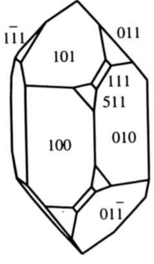
\alpha -Quartz
